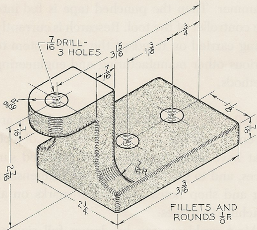
Fig. 10-32. Swivel.*
